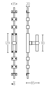
K-FVT110
