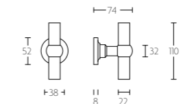
FV22V
