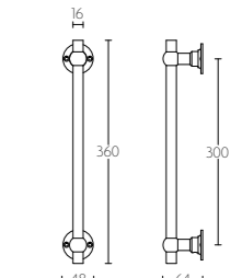
FV360
