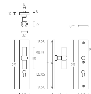
FV22-50
